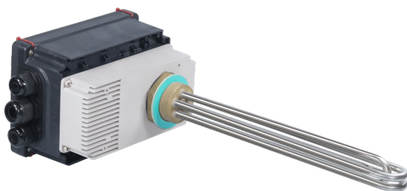
带内置浸入式加热器的温度控制器
