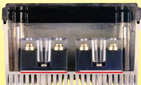
在 Ultimheat 铝壳里的固态继电器的安装示例 (红色为导热膏)
